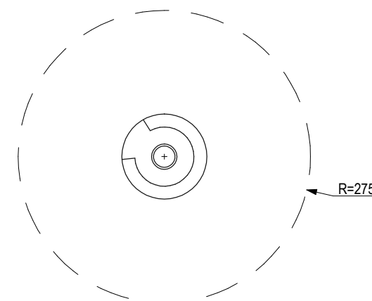
g - karuzala o średnicy 1,6 m z kierownicą
